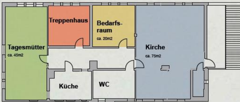
Obergeschoss
