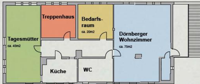
Obergeschoss
